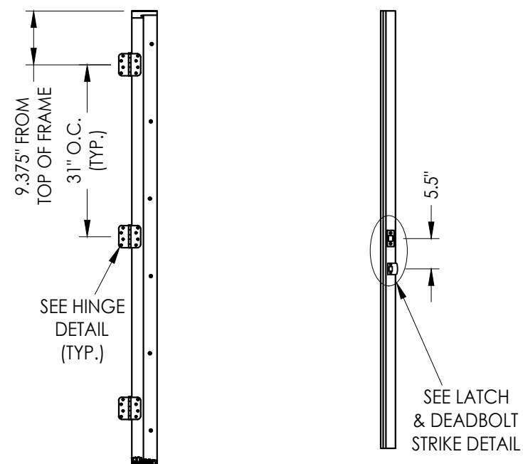
HINGE JAMB
